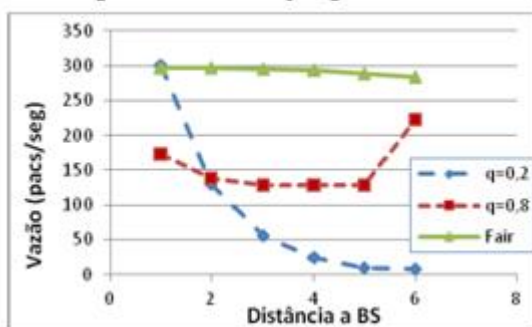
Figura 8 – Vazão na topologia cadeia
