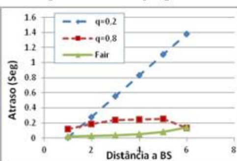
Figura 9 – Atraso na topologia cadeia
